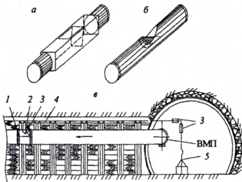
Рис. 1. Устройство для разгазирования тупиковых горных выработок: а, б - схемы устройства; в - схема установки; 1 - патрубок; 2 - клапан; 3 - ролики; 4 - трос; 5 - ручная (электрическая)
