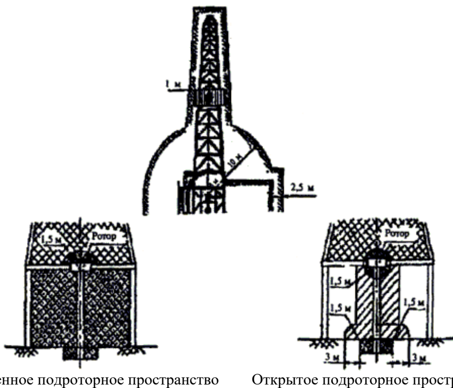
Рис. 2. Буровая установка с укрытием и привыщечным сооружением для бурения скважин на море и месторождениях, содержащих сернистый водород
