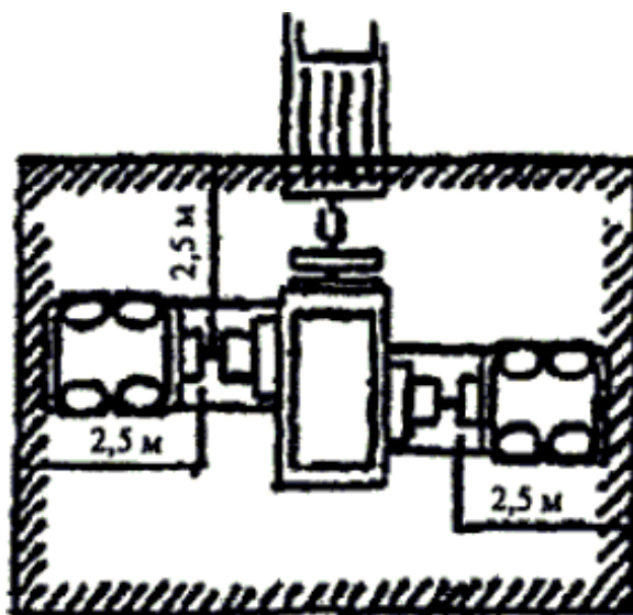
Газовый компрессор
