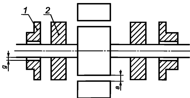
Рисунок 19 — Подшипники скольжения. Случай, когда a < g
