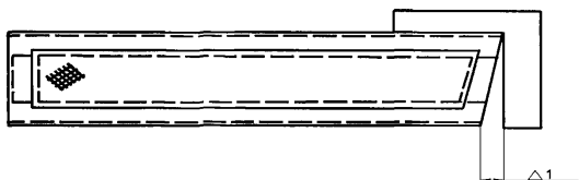
Рисунок 7 Отклонение от перпендикулярности торца рамы, площадки (помоста) относительно боковой поверхности
