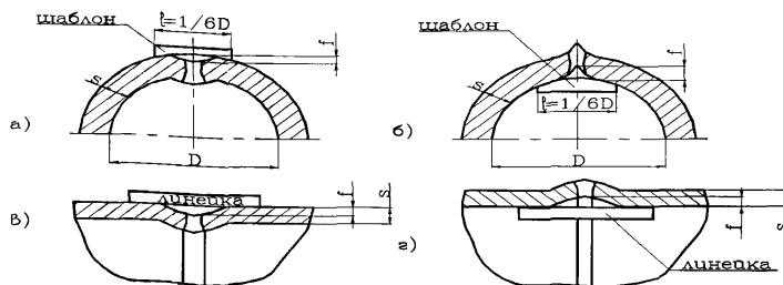
Рисунок 16. Контроль увода кромок продольных (а, б) и кольцевых (в, г) сварных соединений
