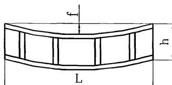
Рисунок 12.Отклонение от прямолинейности конструкции коробчатого сечения
