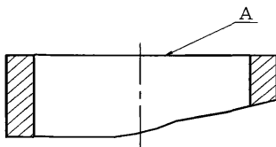
Рисунок 10 Отклонение от перпендикулярности торца А
