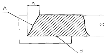
Рисунок 1. Отклонение торца проката от перпендикулярности
