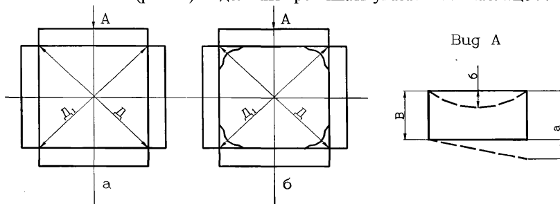
Рисунок 11 Отклонения размеров конструкций коробчатого сечения
