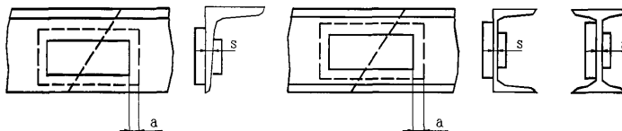
Рисунок 13 Расстояние между сварными швами в противоположных планках
