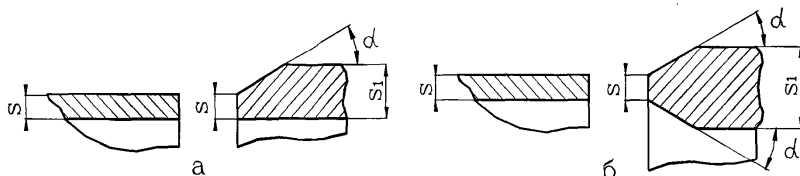
Рисунок 14 Стыковка элементов разной толщины
