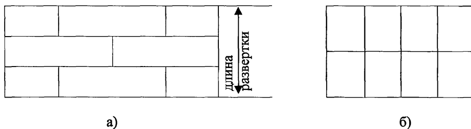
Рисунок 9. Развертка обечаяек
