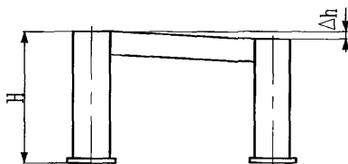
Рисунок 2. Отклонение размеров по высоте рамы, площадки
