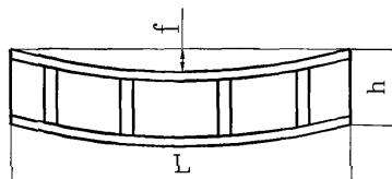
Рисунок 4 Отклонение рамы от прямолинейности (стрела прогиба)
