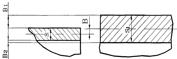
Рисунок 15. Смещение кромок
